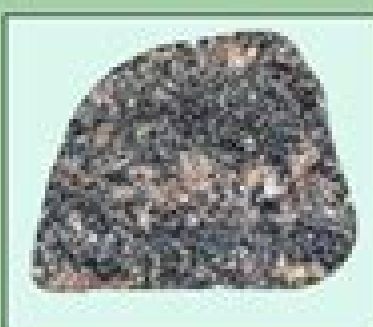
Migmatite
