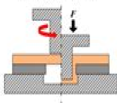
(b) Extensible die
