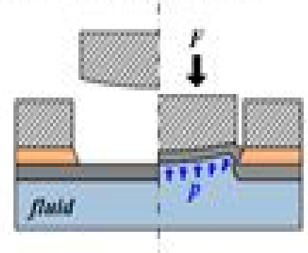
(d) Flat hole clinching
