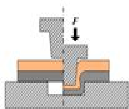
(a) Round flat die
