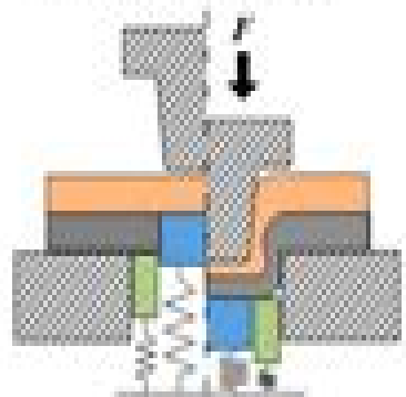
(a) Round flat die
