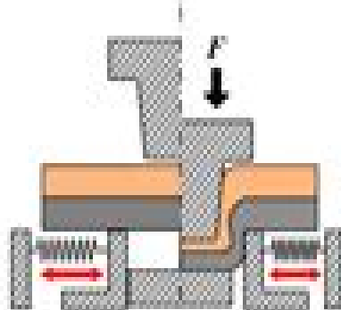
(b) Extensible die
