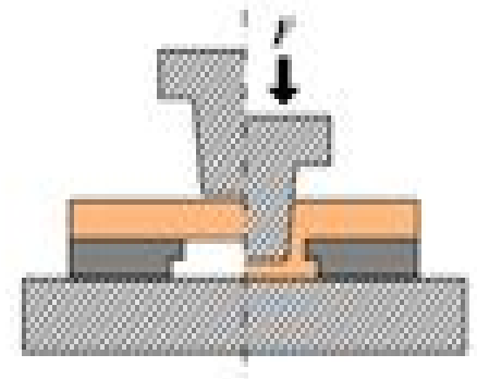
(d) Flat hole clinching
