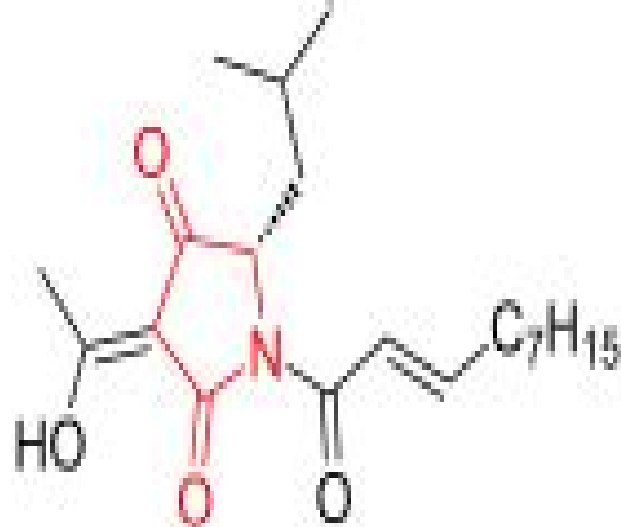
reutericyclin
