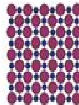
Austenite
