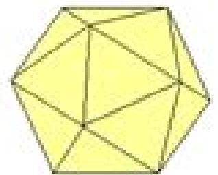
Ikosaeder
