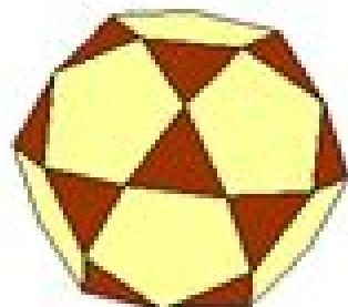
Ikosidodekaeder
