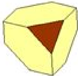
abgestumpftes Tetraeder
