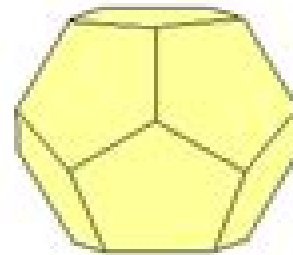
Dodekaeder
