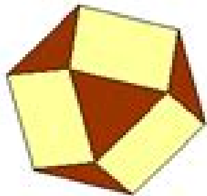
Kuboktaeder
