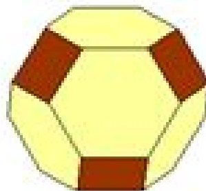
abgestumpftes Oktaeder
