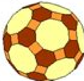
abgestumpftes Ikosidodekaeder
