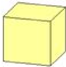
Würfel (Hexaeder)
