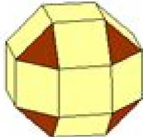
Rhombenkuboktaeder
