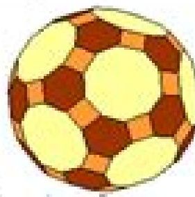
abgestumpftes Ikosidodekaeder
