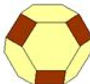
abgestumpftes Oktaeder
