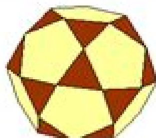
Ikosidodekaeder
