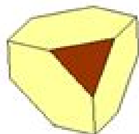
abgestumpftes Tetraeder
