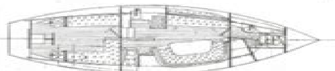
31' MASTHEAD SLOOP
