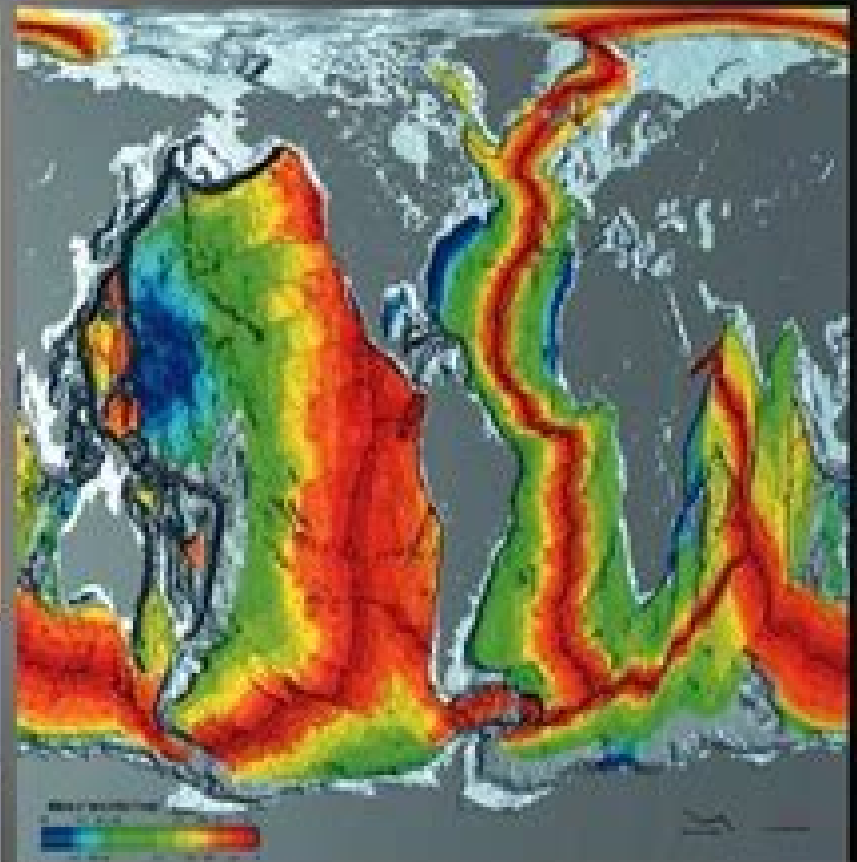
Возраст земной коры
