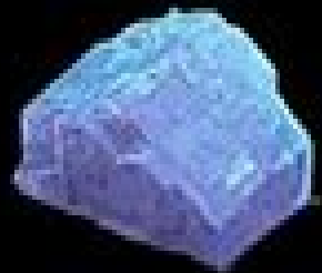
Pezzotaite
