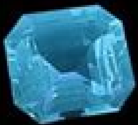
Beryl Morganite
