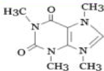
CAFFEINE
