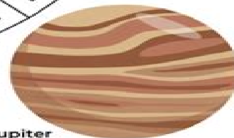
Jupiter
