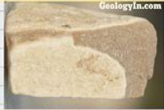
Mudstone
