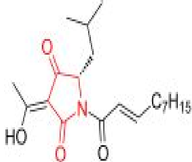
reutericyclin
