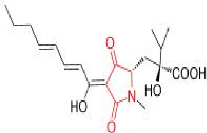
harzianic acid
