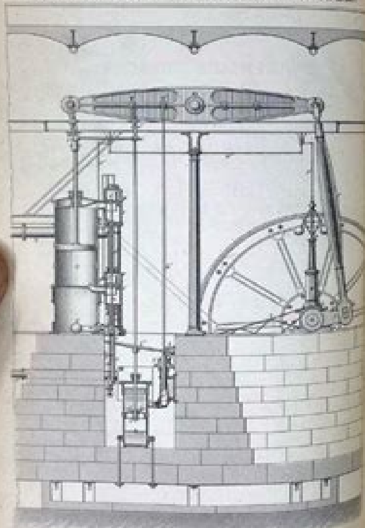
Longitudinal Section
