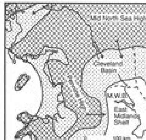
(d) Mid Jurassic
