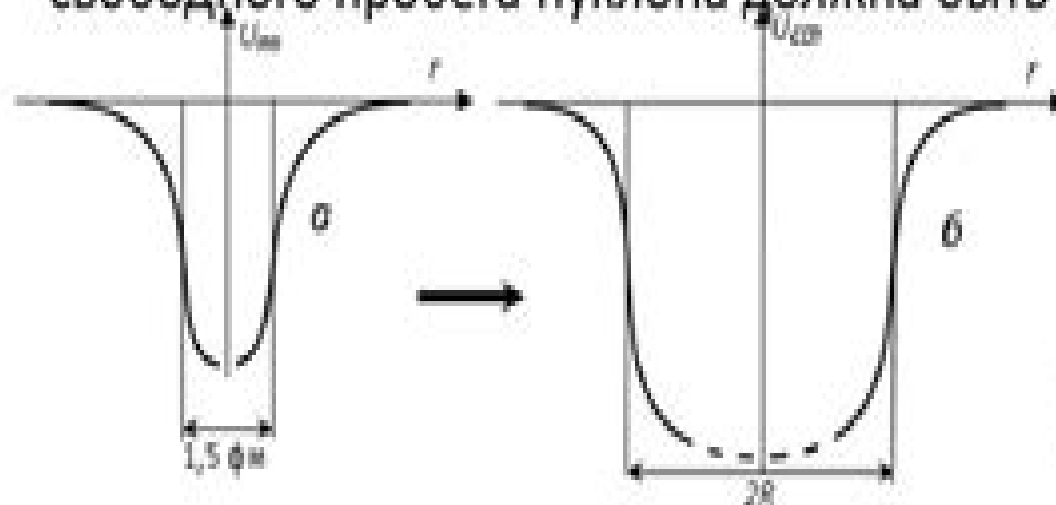
Нуклон-нуклонный потенциал (а) потенциал самосогласованного поля (б)
