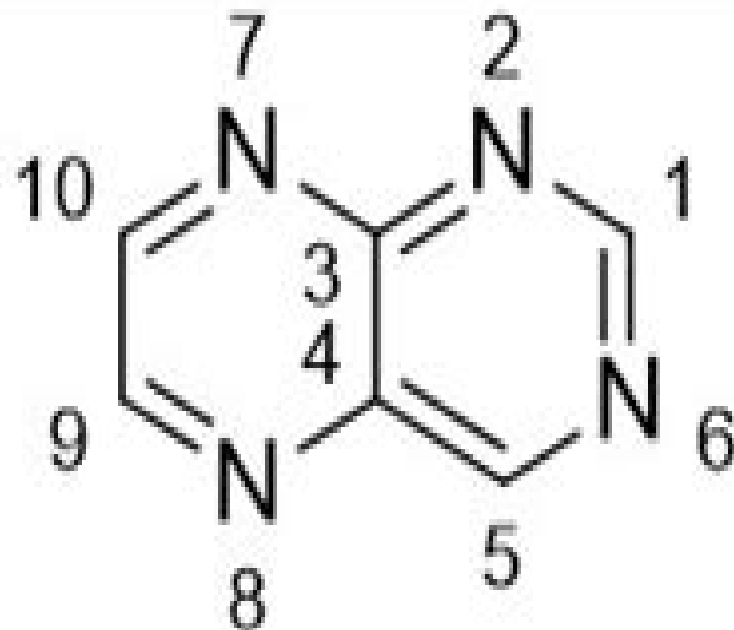
Pteridine
