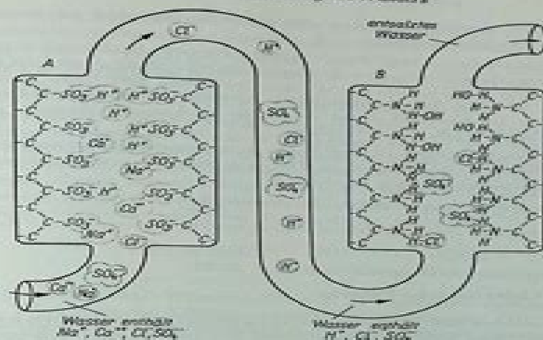
Abb. 15-1. Entfernen von Ionen aus Wasser durch Kationenaustauscher und Anionenaustauscher.
