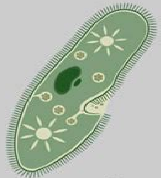
Paramecium
